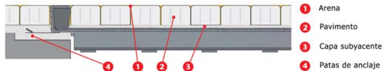
Sección puesta en obra
