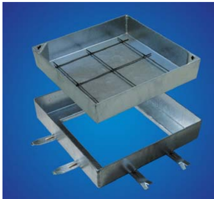
Detalle del modelo rellenable Urban, en acero galvanizado
