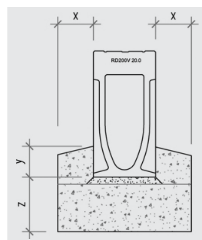
Esquema sección ACO Monoblock tipo "I"
