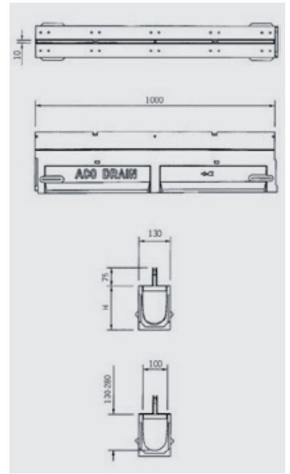
Sección canal Brickslot.
