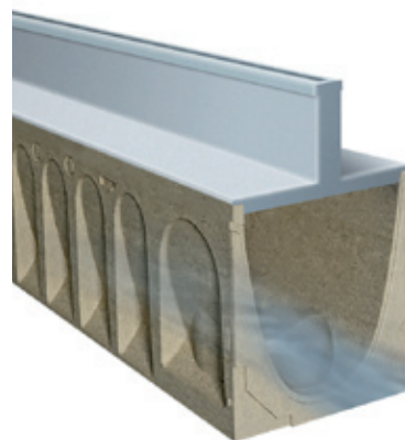
Sección de la instalación del Brickslot®
