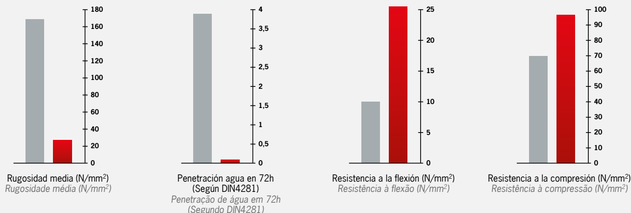
Comparación entre características del hormigón tradicional con el hormigón polímero. Comparação entre características do betão tradicional com o betão polímero.
