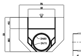
Tapa Universal · Tampa Universal
