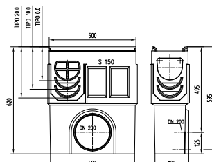
Plano sumidero Elementos técnicos do sumidouro
